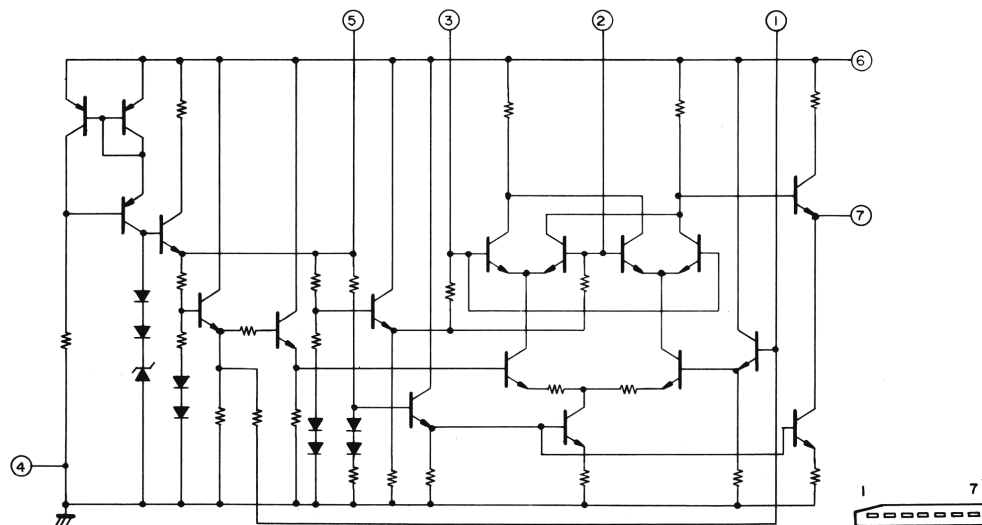
IC3 AN612
